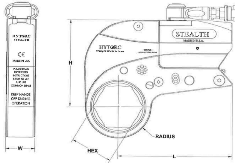
寸法図
